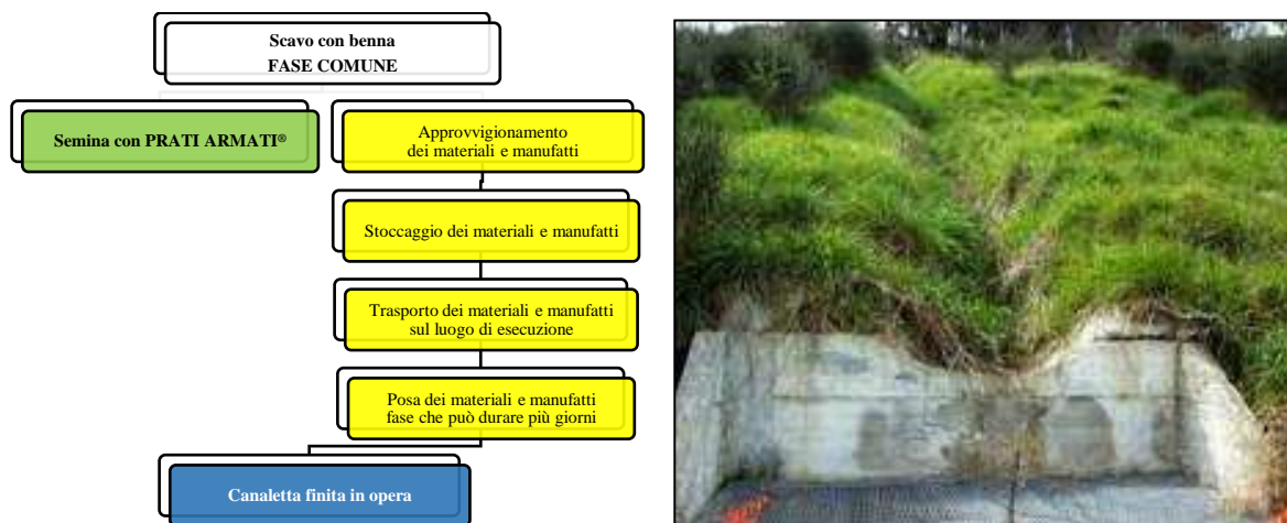
Figura 3. Confronto della complessità realizzativa di canalette tradizionali raffrontate alla semplicità di canalette inerbite.
