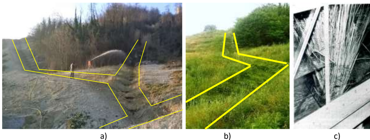
Figura 5. RFI S. Vittoria d'Alba Canalette realizzate direttamente sul tal quale con piante allettanti frammiste a piante assurgenti, elastiche, tenaci e particolare della dissipazione dell'energia idraulica da parte di queste ultime.
